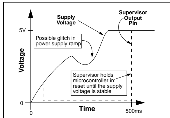
FIGURE 1: POR FUNCTION
